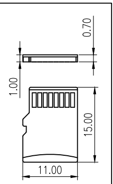
T-Flash
