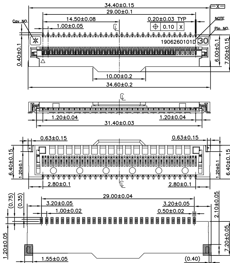
P.C.B Layout
