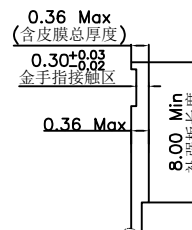
APPLICABLE FPC RECOMMENDED DIMENSION 蓝白裸线（不接地）
