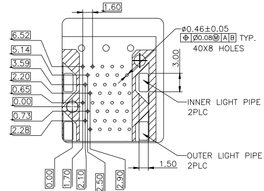
DETAIL H 2:1
