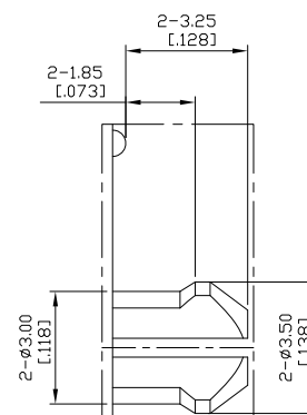
DET.A SCALE 2:1
